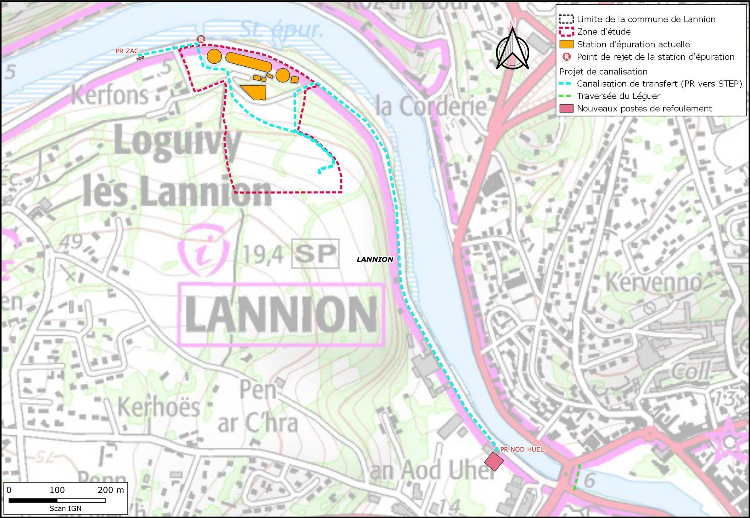
Figure 2 : Plan de projet des nouvelles canalisations de transfert entre les nouveaux PR (Nod Huel et ZAC) et la future STEP
