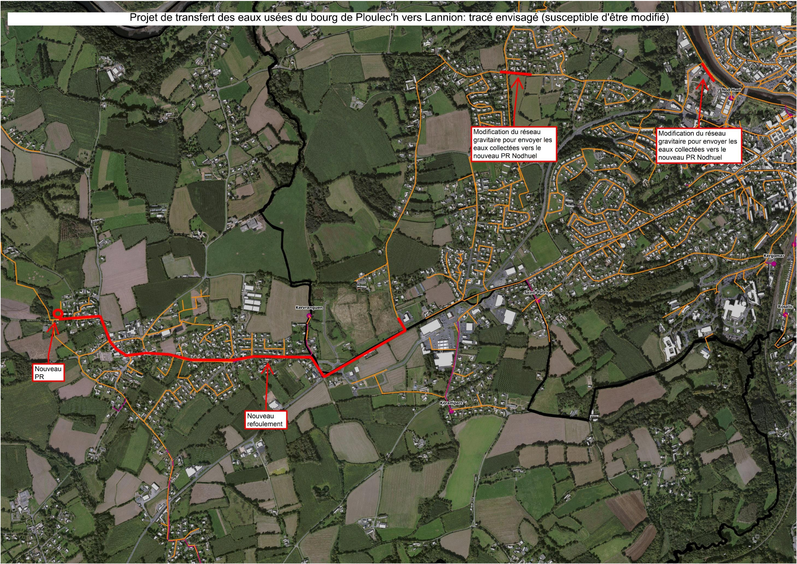
Figure 3 : Plan de projet du réseau de transfert des eaux usées du bourg de Ploulec'h vers le PR Nod Huel
