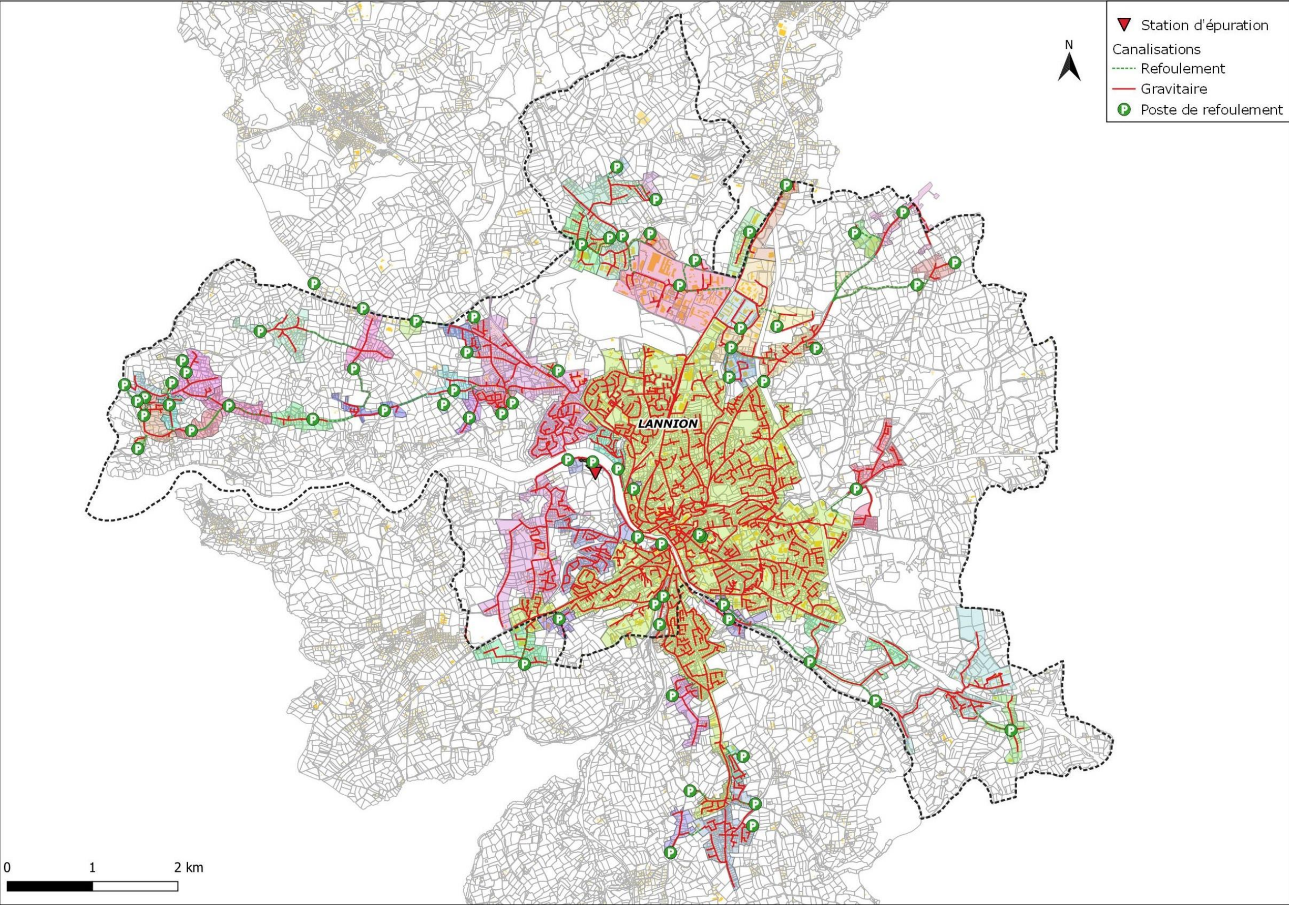
Figure 1 : Plan du réseau de collecte raccordé à la station d'épuration de Lannion
