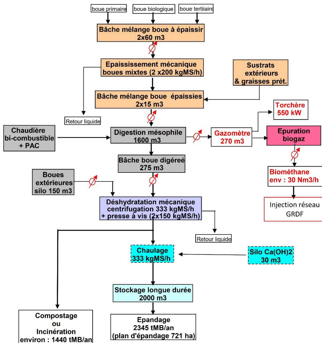
Figure 5 : Synoptique de la future filière Boues
