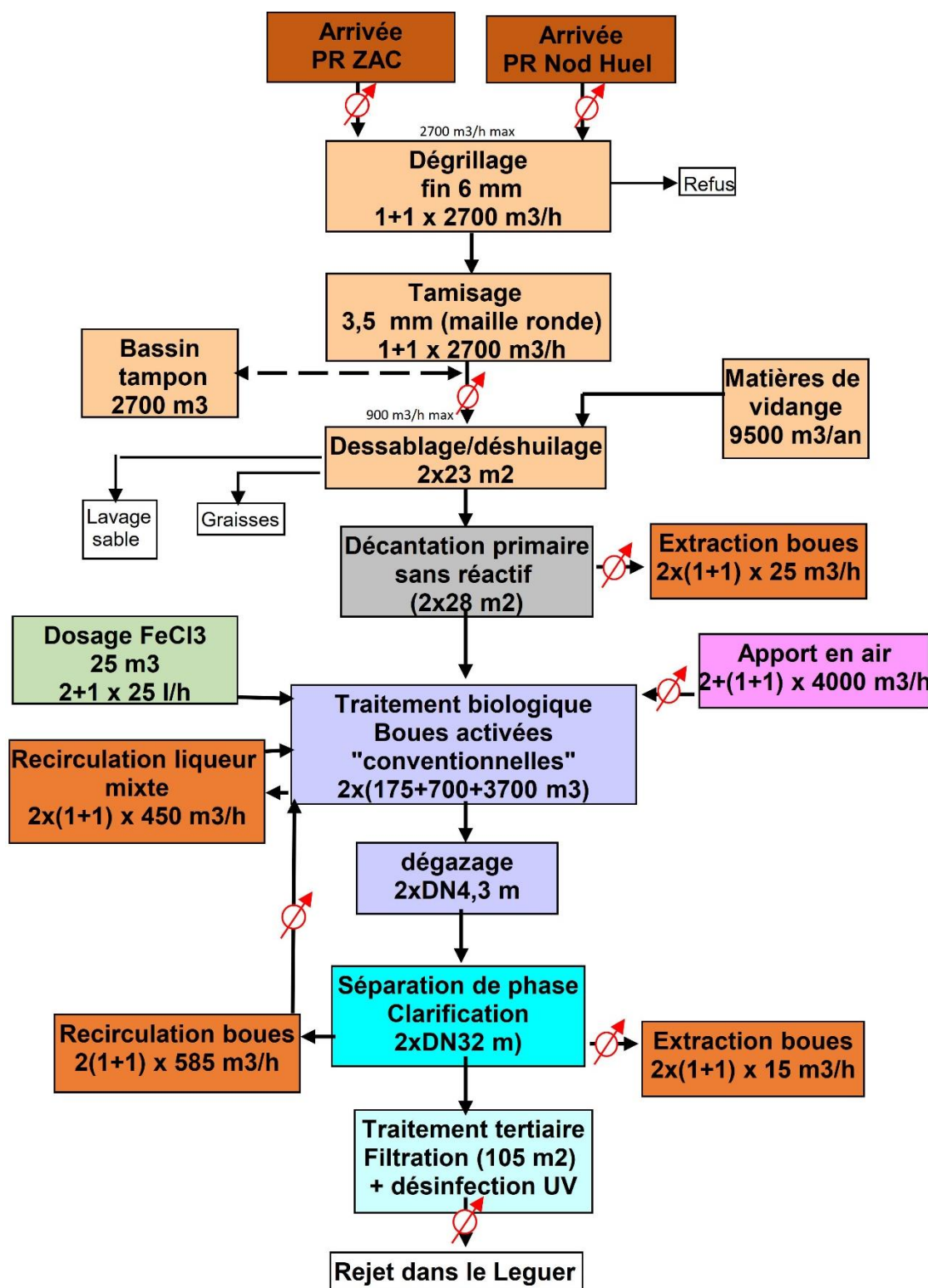
Figure 4 : Synoptique de la future filière Eau
